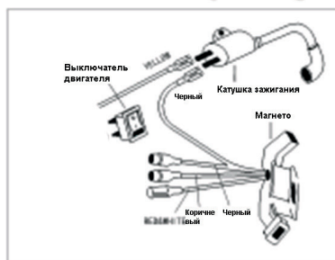
Схема зажигания
